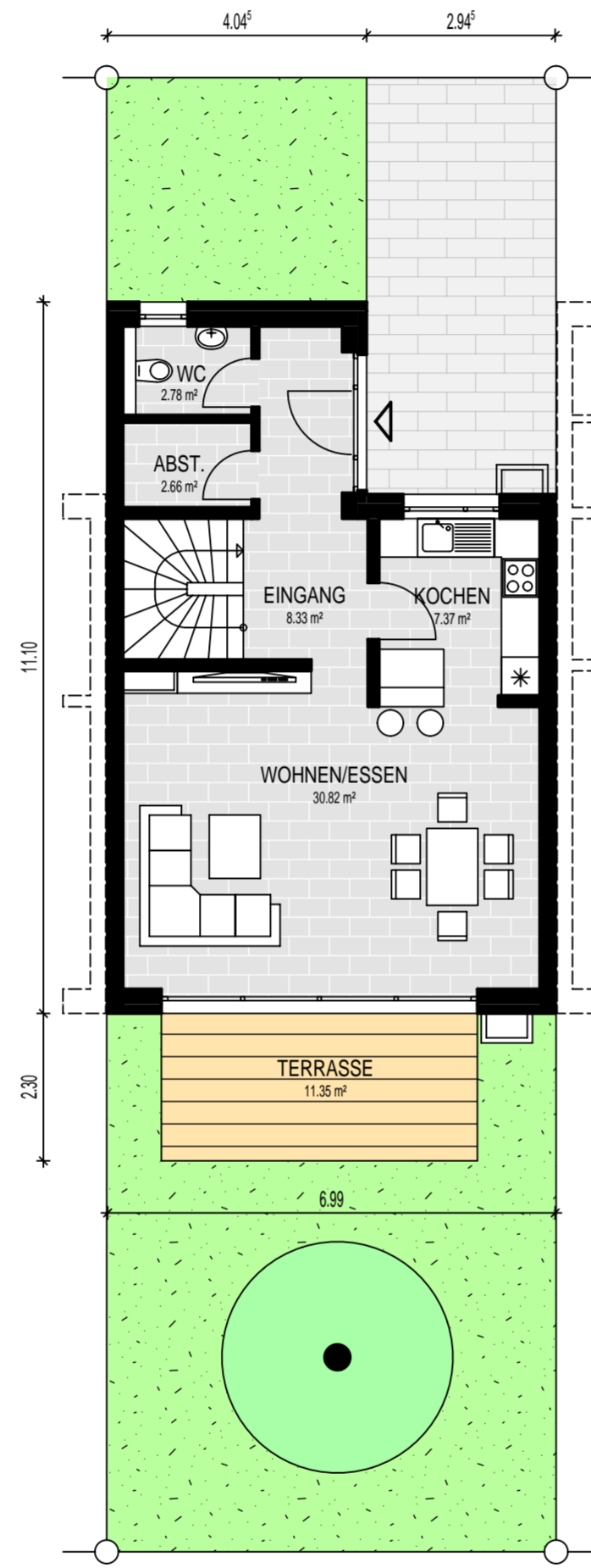
ERDGESCHOSS
