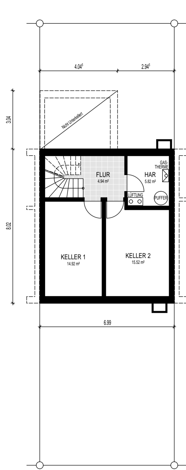
KELLERGESCHOSS
