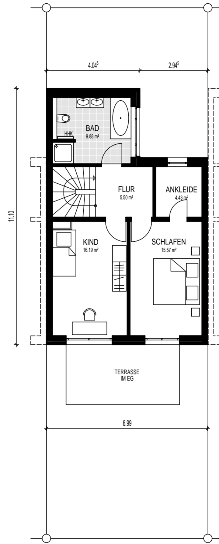
OBERGESCHOSS
